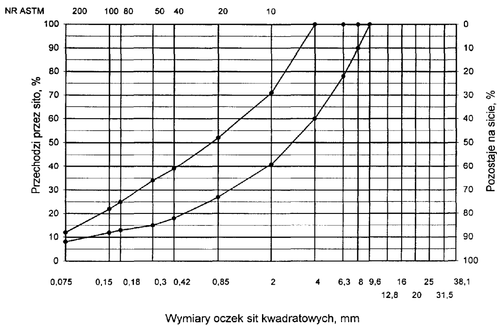
Rys. 2. Krzywe graniczne uziarnienia mieszanki mineralnej BA od 0 do 16mm, od 0 do 12,8 mm do warstwy ścieralnej nawierzchni drogi o obciążeniu ruchem KR1 lub KR2 Rys. 3. Krzywe graniczne uziarnienia mieszanki mineralnej BA od 0 do 8mm, od 0 do 6,3 mm do warstwy ścieralnej nawierzchni drogi o obciążeniu ruchem nawierzchni drogi o obciążeniu ruchem KR1 lub KR2
