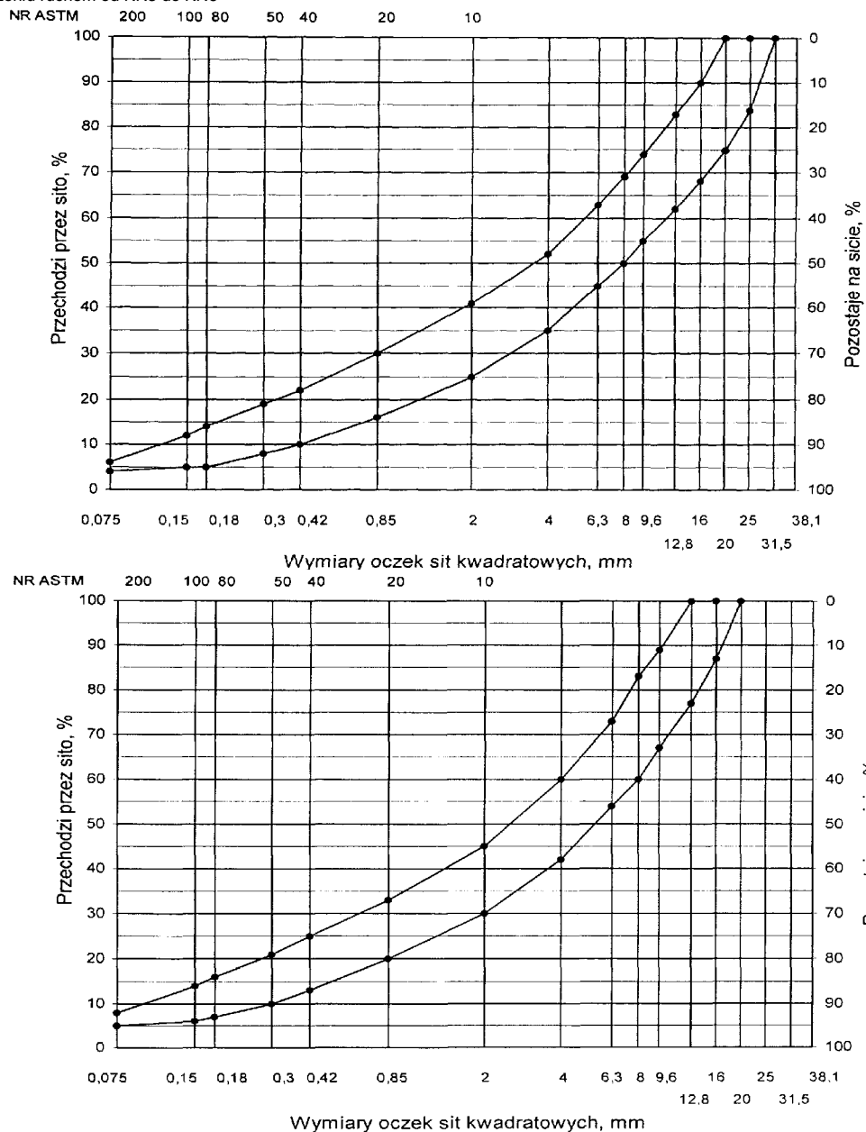
Rys. 11. Krzywe graniczne uziarnienia mieszanki mineralnej BA od 0 do 25 mm do warstwy wiążącej, wyrównawczej i wzmocniającej nawierzchni drogi o obciążeniu ruchem od KR3 do KR6
