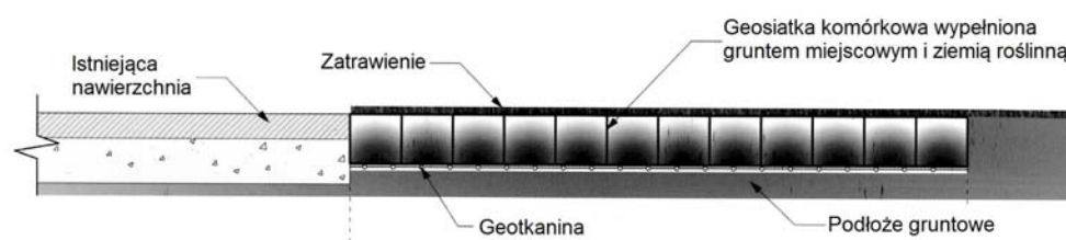
Rys. 14. Przykładowe przekroje poprzeczne utwardzonego pobocza, wykonanego przy użyciu geosiatki komórkowej
